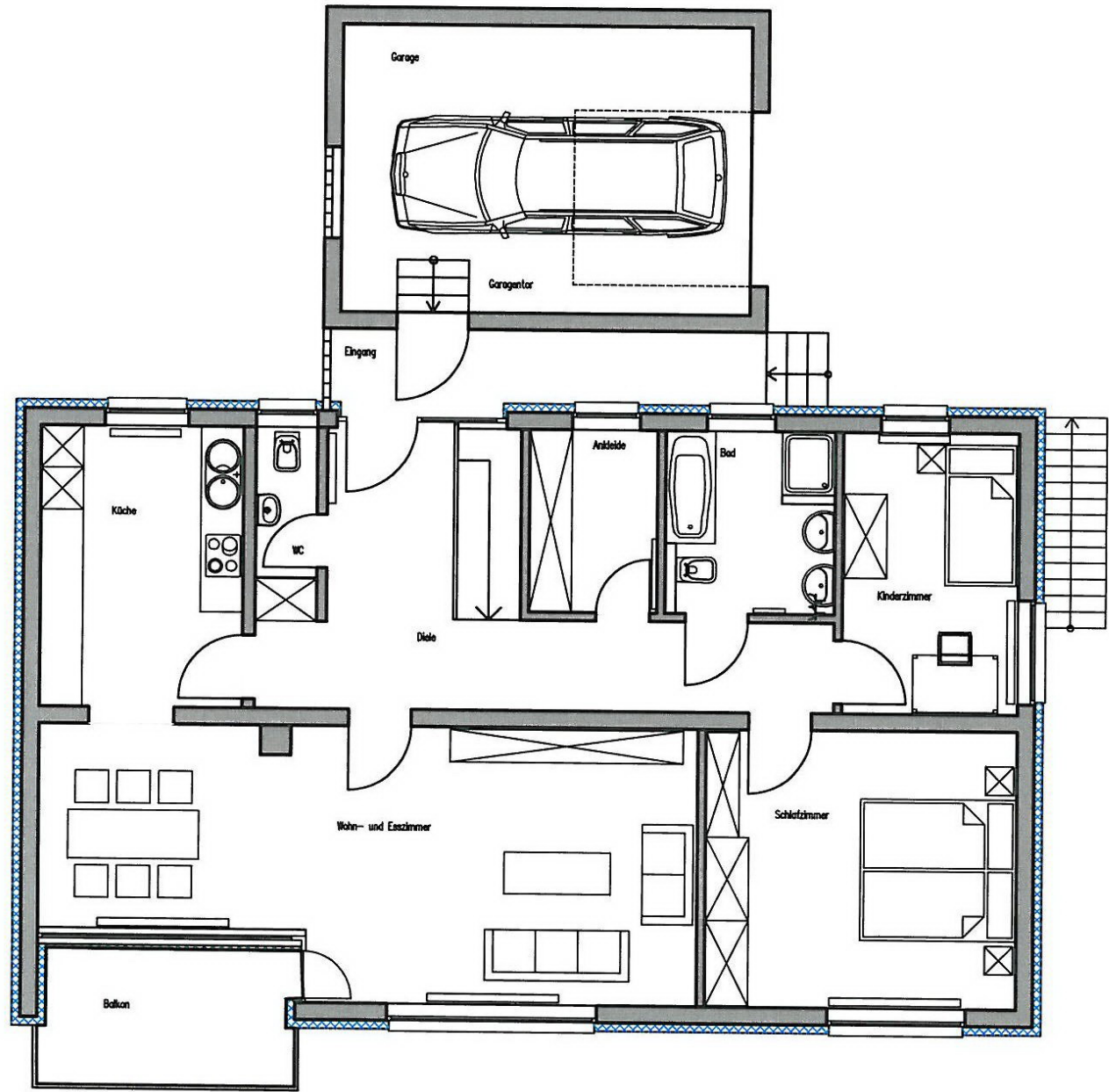
Grundriss Erdgeschoss
