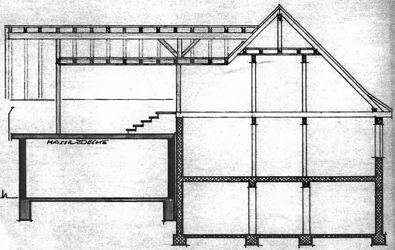
LÄNGSSCHNITT
