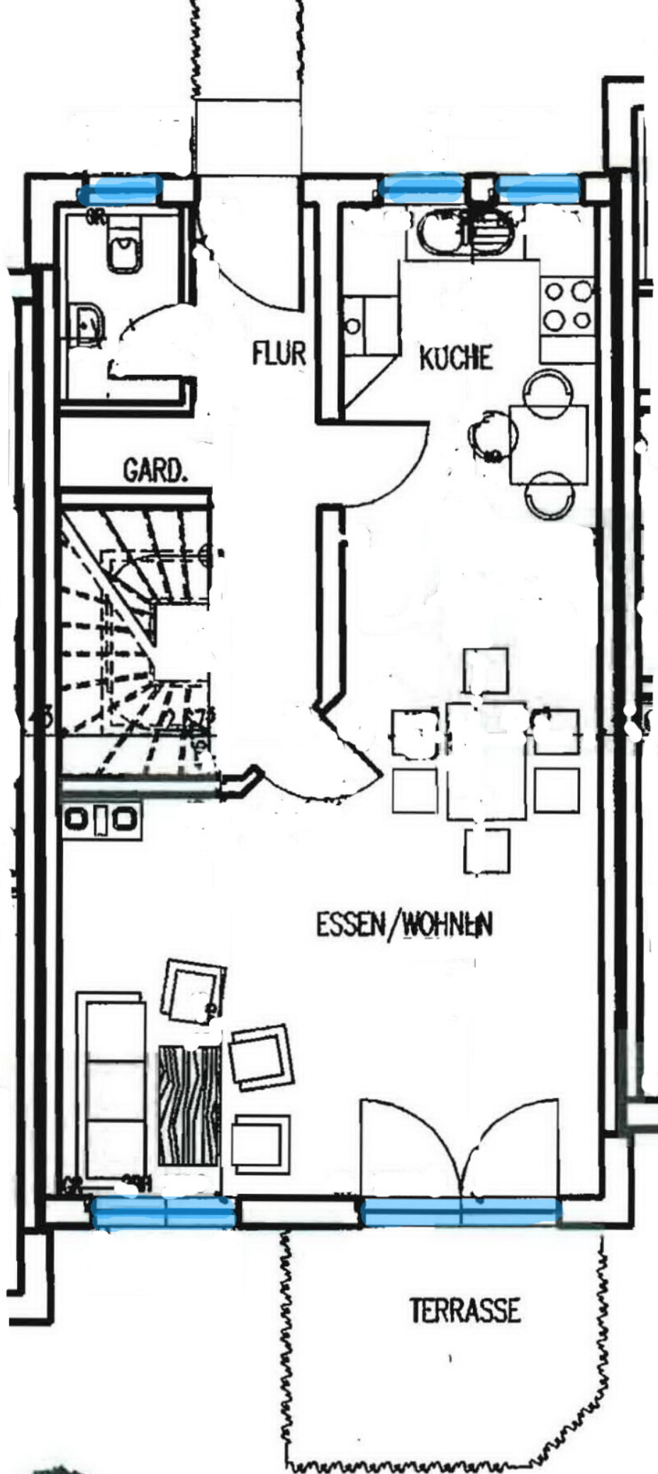
Erdgeschoss
