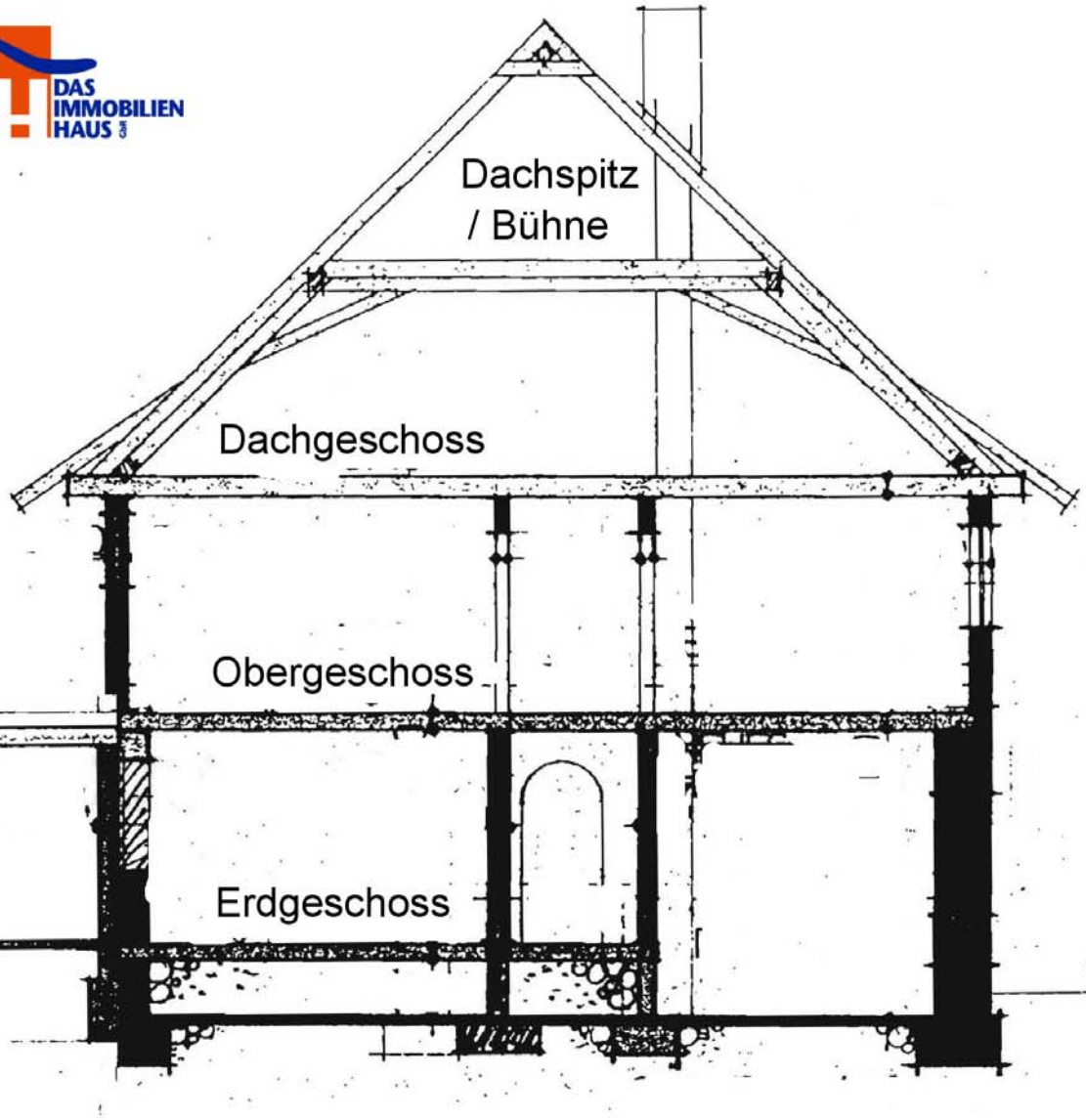
Schnitt
