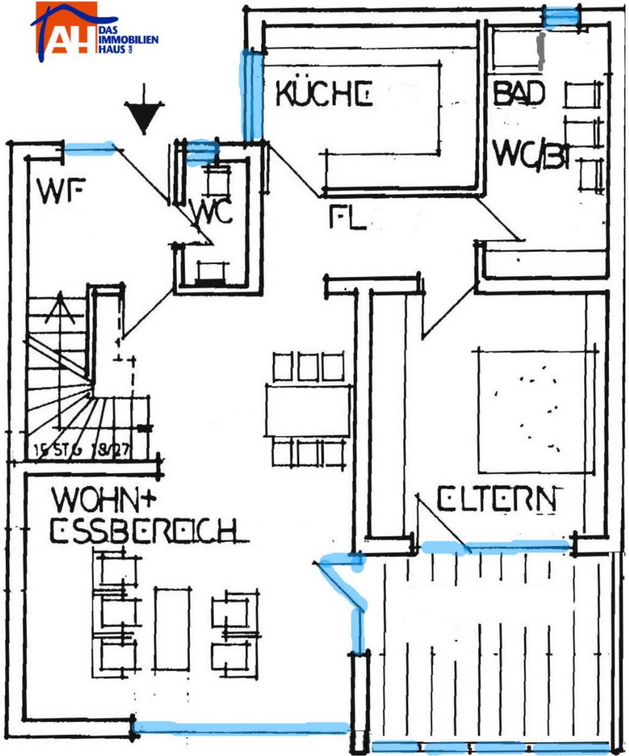
Erdgeschoss
