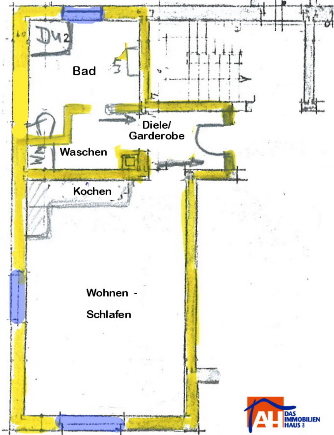
Wohnungsgrundriss (Souterrain)
